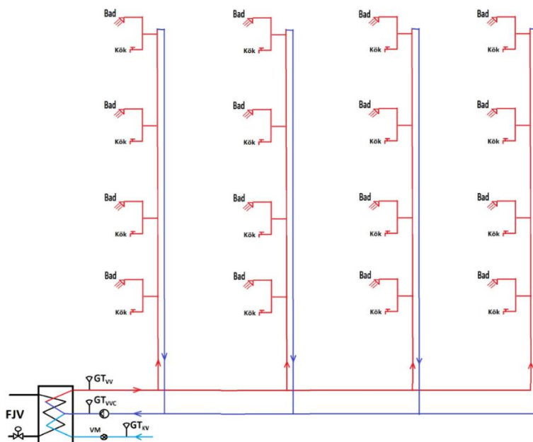
Figur 3 Principskiss varmvatten/varmvattencirkulationssystemen
