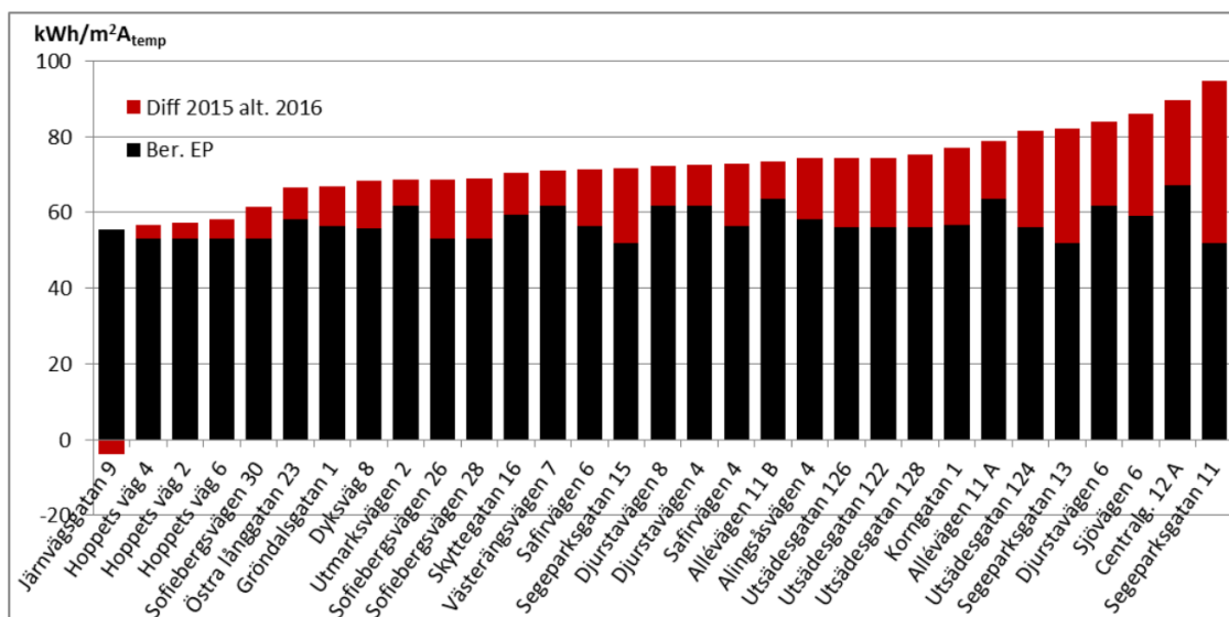
Figur 2 Uppmätt normalårskorrigerad energiförbrukning för fjärrvärmvärmda Kombohus Bas 2016 jämfört med beräknad (kWh/m 2 ). Hela stapelhöjden avser uppmätt energiförbrukning. Skillnaden mellan beräknad och uppmätt energiförbrukning framgår av differensen. För stapeln längs till vänster är uppmätt energiförbrukning något mindre än beräknad.
