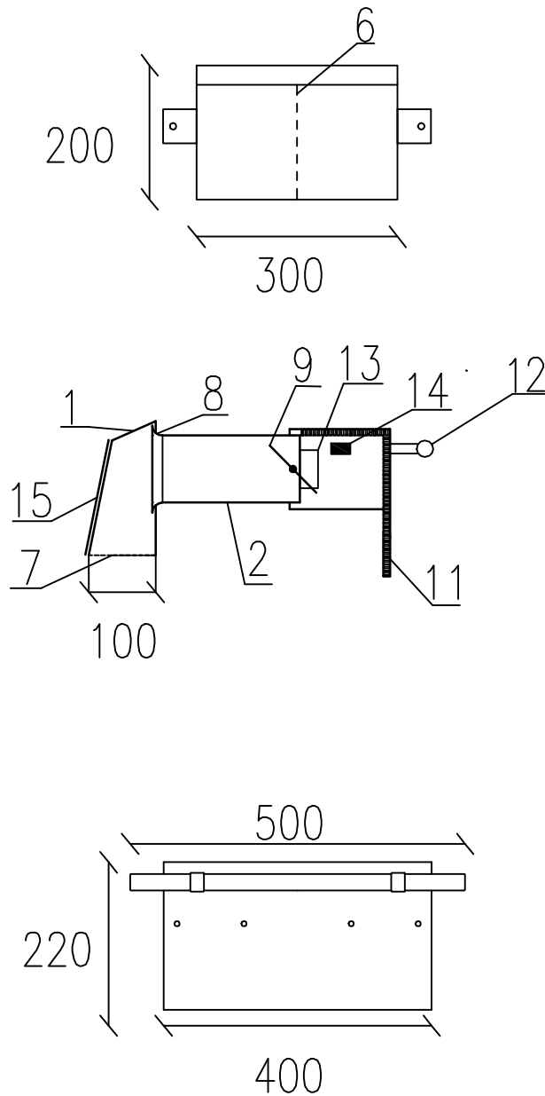
FIG 2 AUDIC AB 1:10 SPISKÅPA UTELUFTSDON, INOMHUSDEL DIDRIK AURENIUS 20200202
