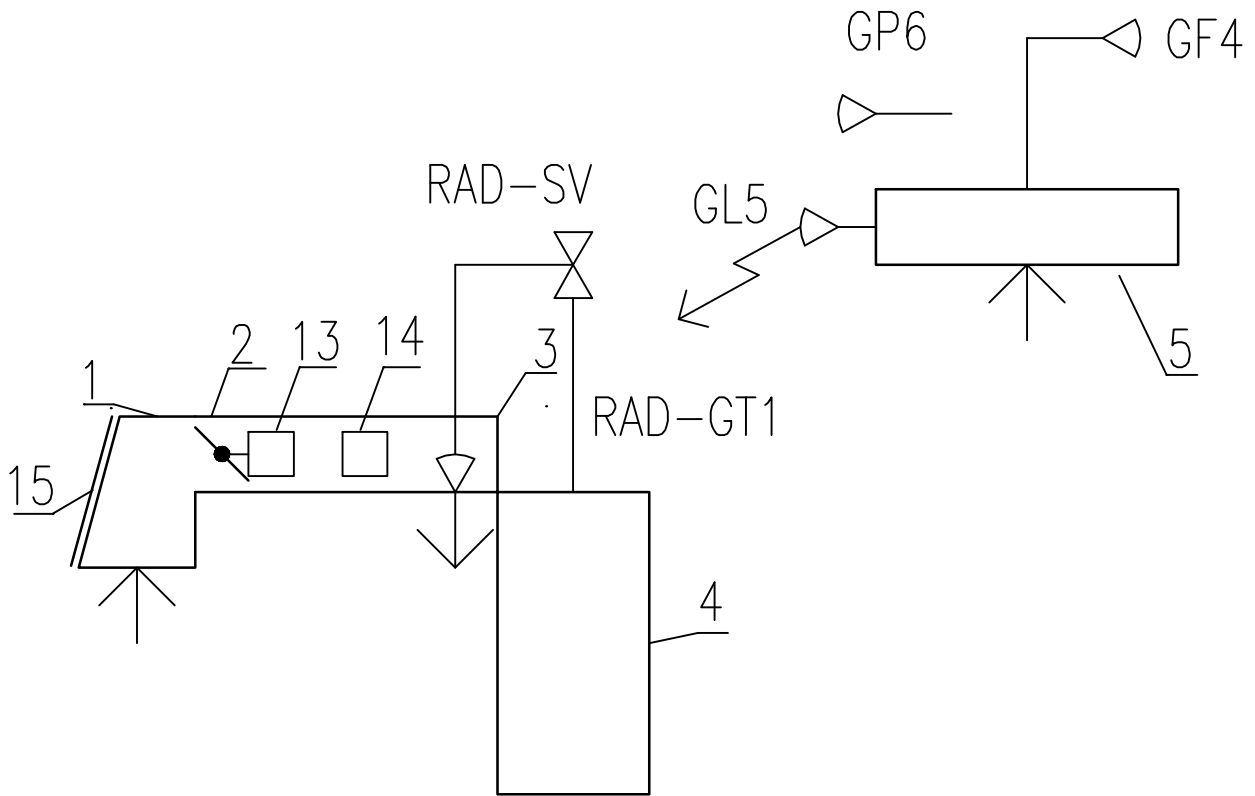
FIG 3 AUDIC AB SPISKÅPA PRINCIPSCHEMA DIDRIK AURENIUS 20200202
